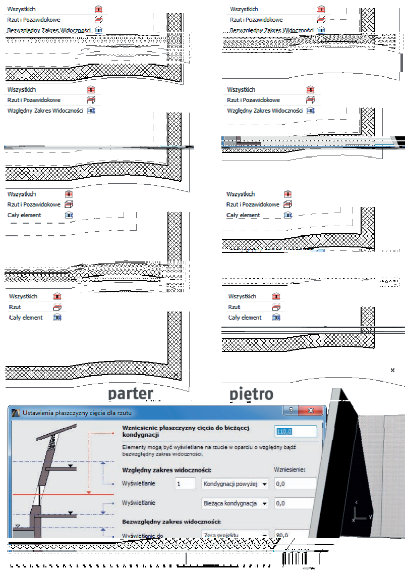
Rysunek 9.32. Przykład pokazujący najważniejsze różnice w wyświetlaniu symbolu zależnie od ustawień Płaszczyzny cęcia dla rzutu — na rysunku ten sam zestaw trzech Ścian pochyłych w czterech różnych układach opcji widoczny na dwóch kolejnych kondygnacjach (parter, piętro)
